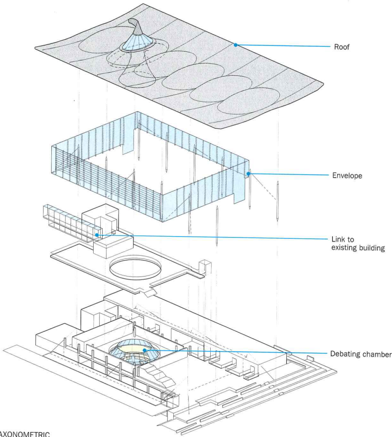
AXONOMETRIC
